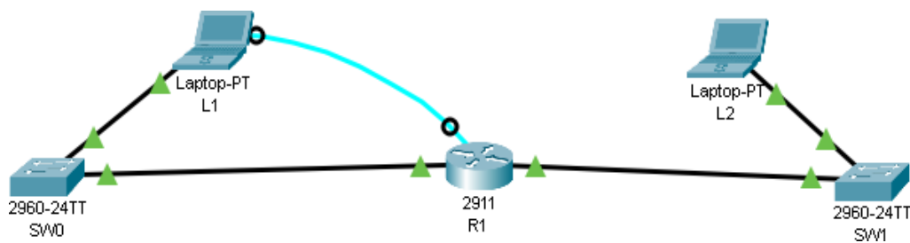
Figura 1. Diagrama de Red MOBIL BOTICA
